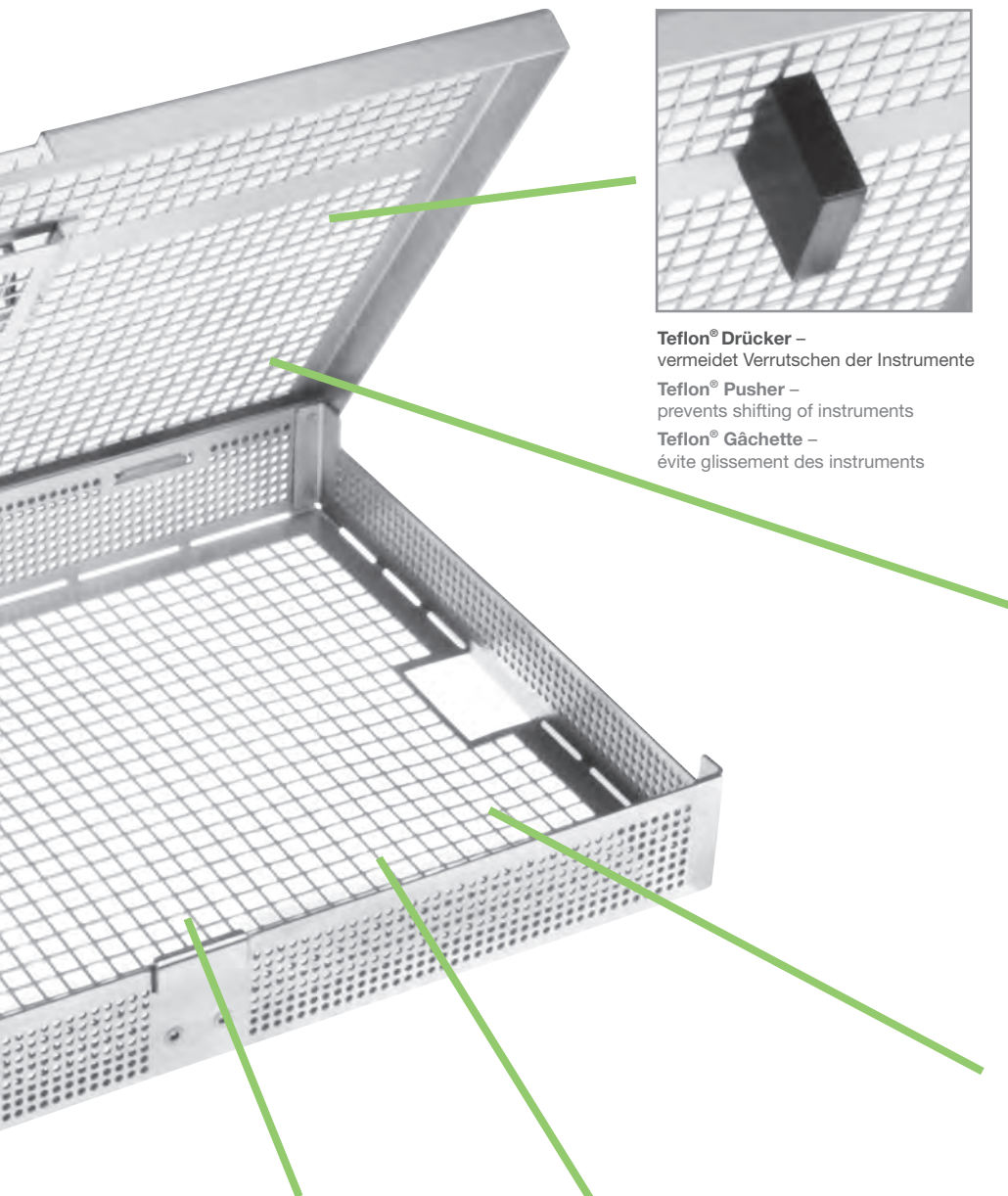
Silikonleiste – fixiert die Instrumente perfekt Silicone band – perfect fixation of the instruments Joint en silicone – fixation optimale des instruments
